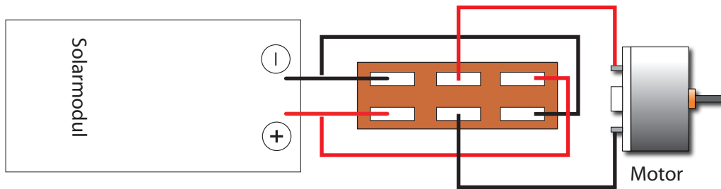
Schiebeschalter 2xUM/ ON-OFF-ON
